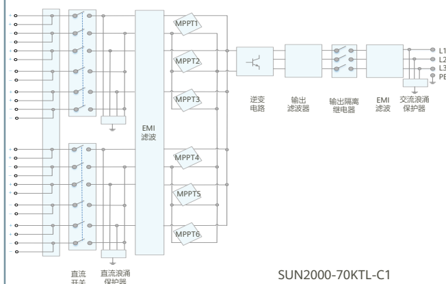
电路框图
