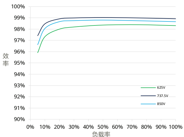
效率曲线
